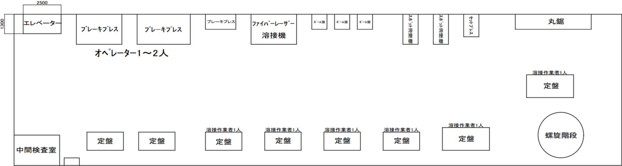
2F工場配置図
